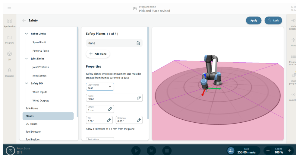
図 1.5: 安全平面を表示する PolyScope X 画面。
