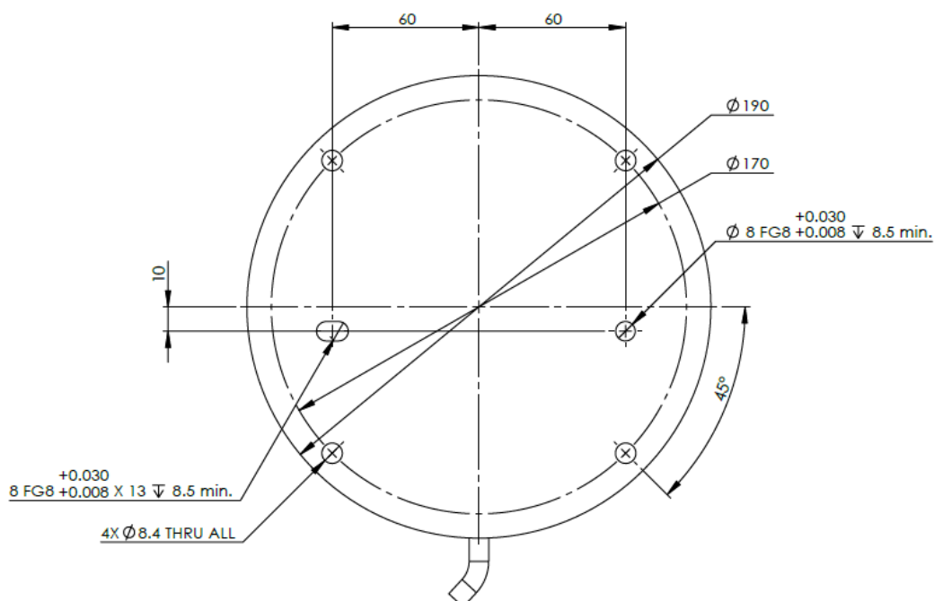
1.1: ロボットベースの底面図
